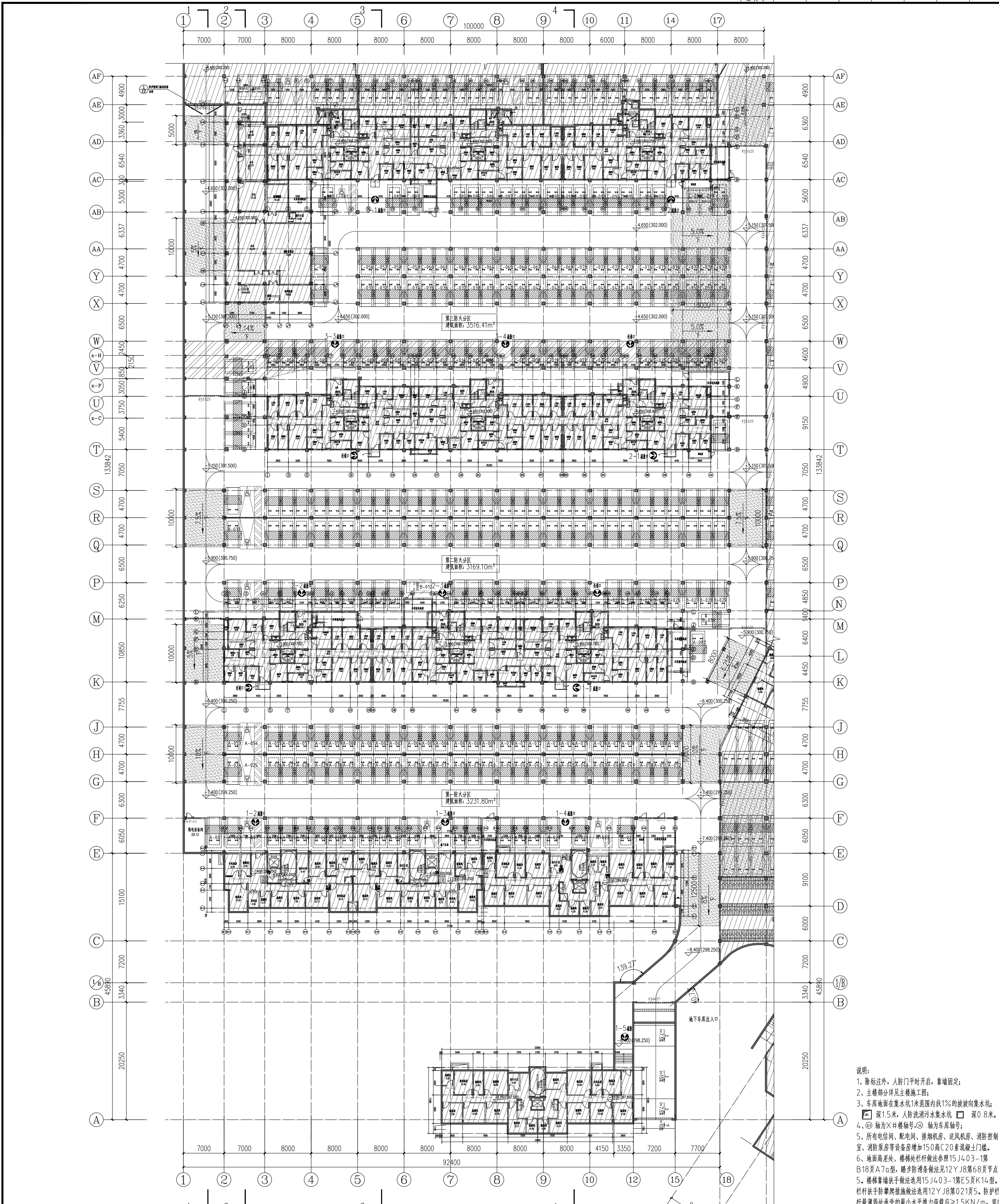
地下一层组合平面图 1:300
